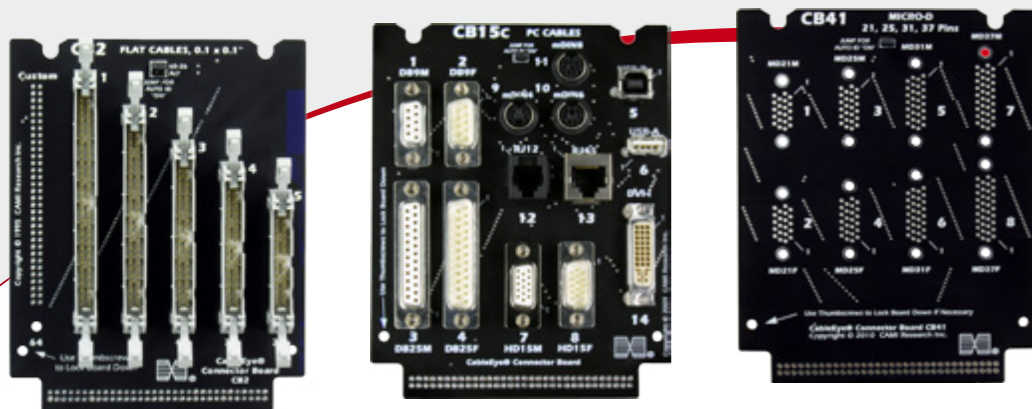
Abb. 1: Für nahezu unbegrenzte Stecker-Typen können CableEye Adapterplatinen mit Gruppen von Anschlüssen bestückt werden oder zur Anpassung frei bleiben. Im Bild sind Konfigurationslösungen für USB-, Sub-D-, Nano-D-, Micro-D-, IDC-Kabelmontage-Buchsen und mehr dargestellt.
